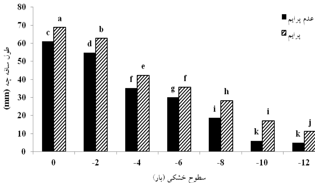
نمودار ۵- مقایسه میانگین اثر متقابل پرایم × تنش بر صفت طول ساقه بچه گلرنک تحت تنش خشکی.
